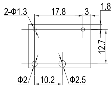
安装尺寸图
