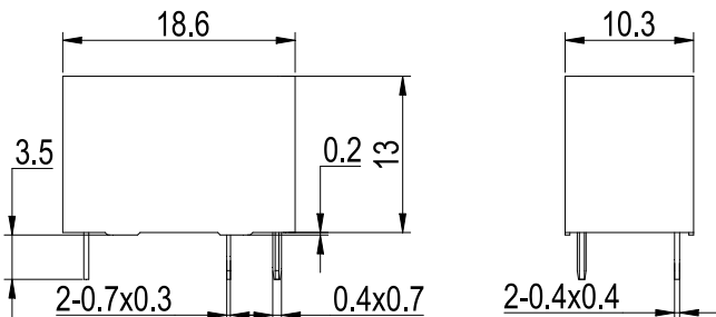
外形尺寸图
