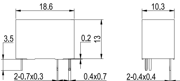
外形尺寸图
