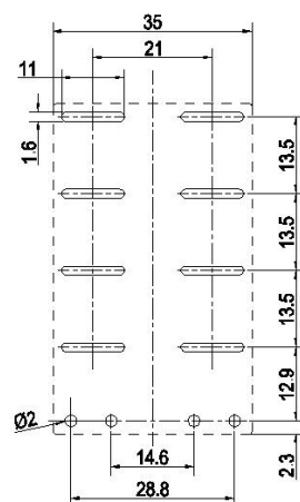
安装尺寸图 (底视图)
