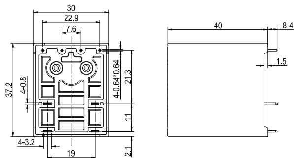
外形接线图
