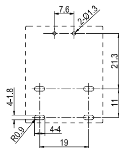
安装尺寸图 (底视图)
