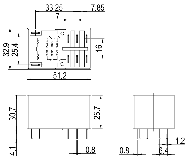
外形尺寸图
