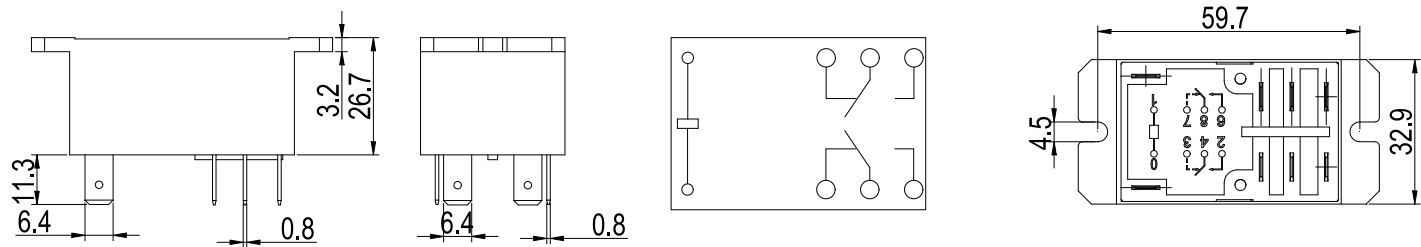
外形尺寸图
