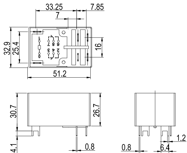
外形尺寸图
