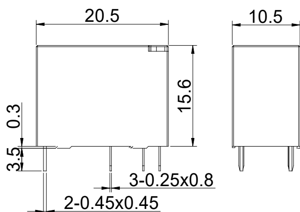
外形尺寸图
