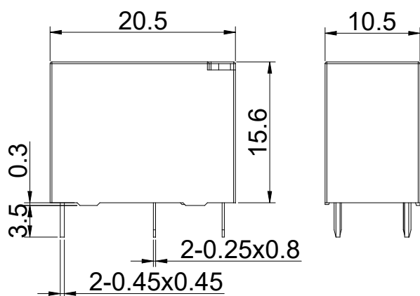
外形尺寸图
