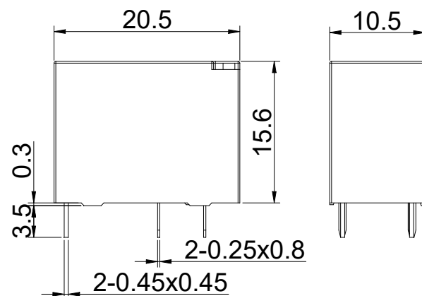
外形尺寸图
